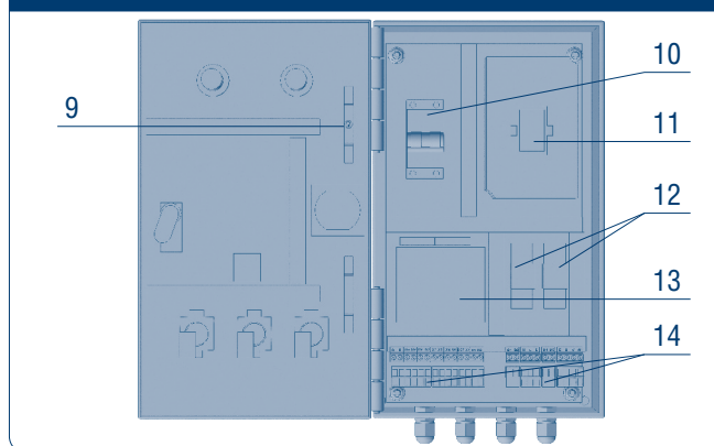
Рис. 2. Открытое положение
