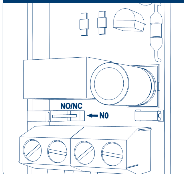
Рис. 43.2. Фотоэлемент. Положение переключки — NO
