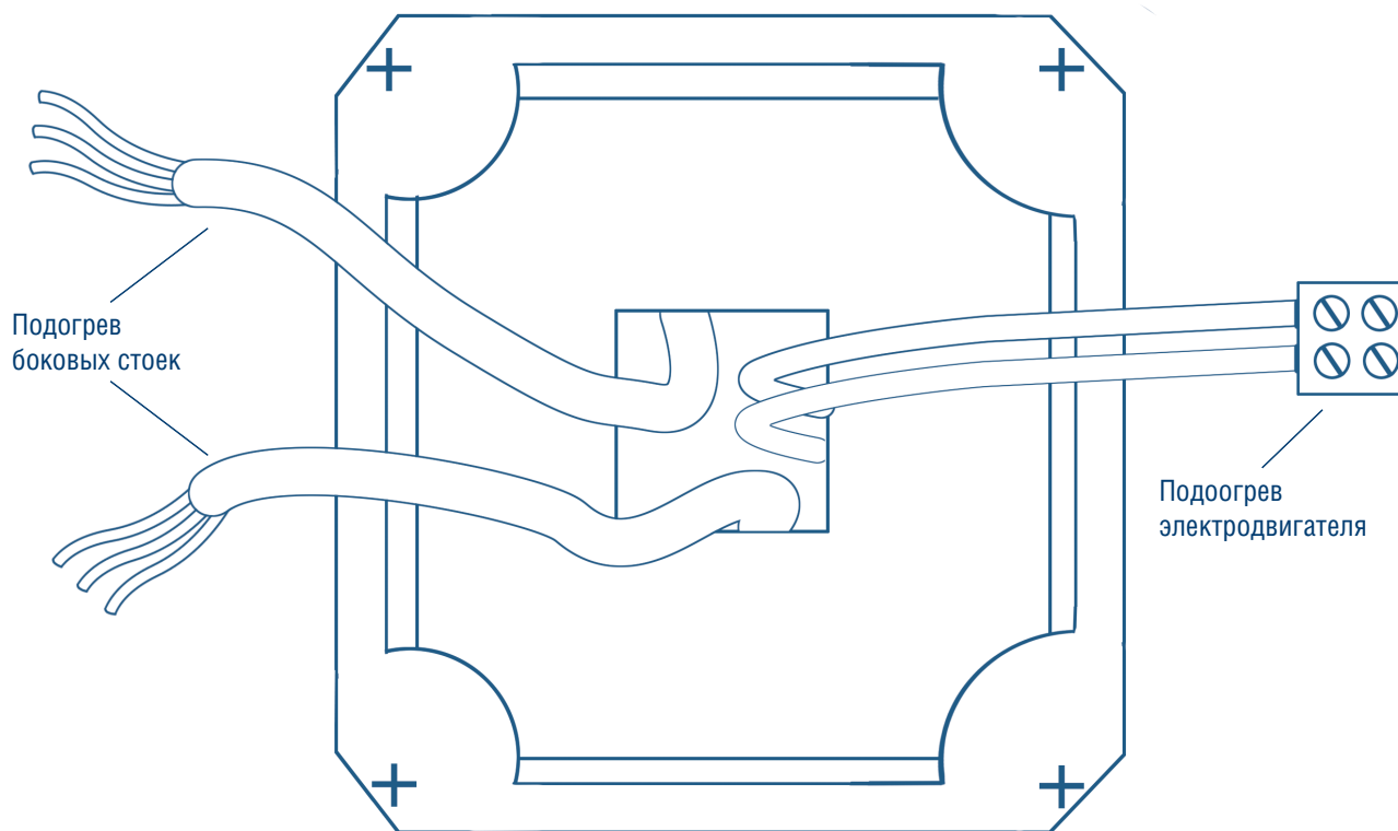
Рис. 39. Схема подключения
