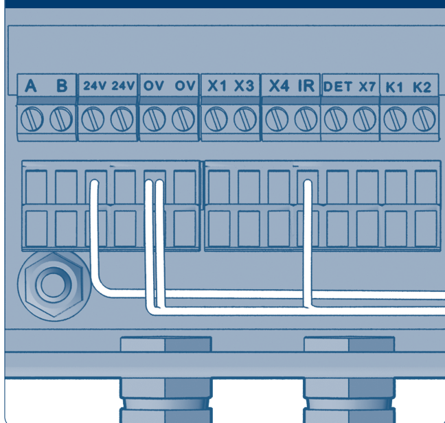
Рис. 31. Монтажная схема
