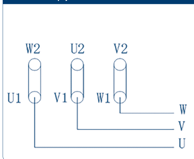
Рис. 4. Схема «треугольник»
