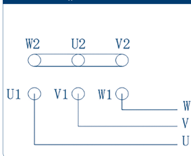
Рис. 5. Схема «звезда»
